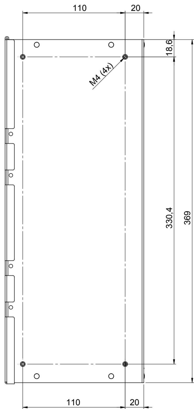
Seitenansicht
